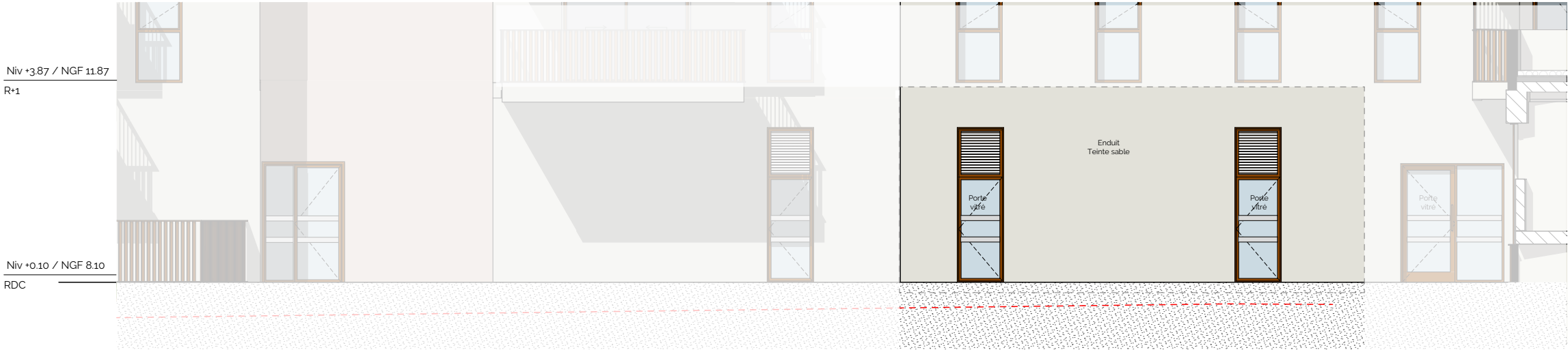
C - Façade Nord-Est en coeur d'îlot
